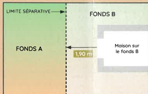
Vue droite
